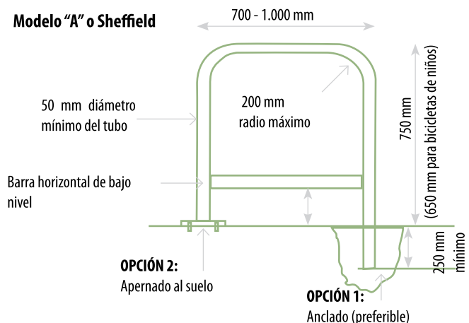
Gráfico 22. Modelo A
