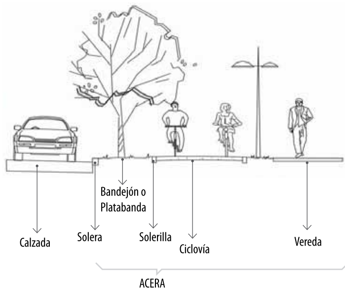
Gráfico 26. Términos básicos
